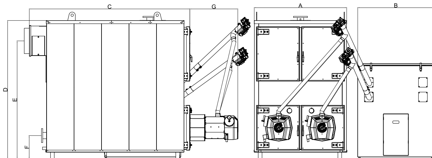
MAXPelL GL 450 dwa palniki
