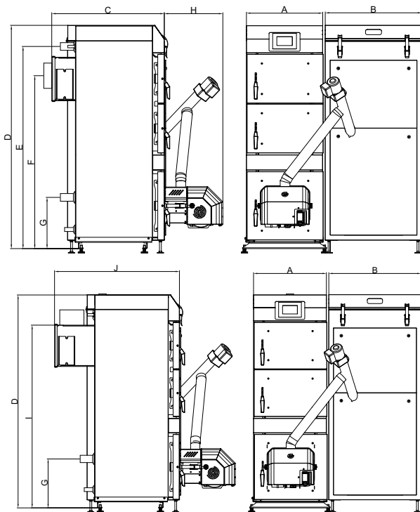
Kocioł z wyprowadzeniem spalin do góry
