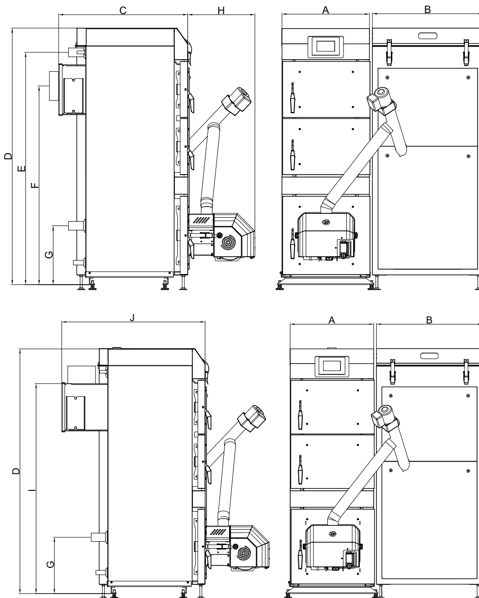
Kocioł z wyprowadzeniem spalin do góry
