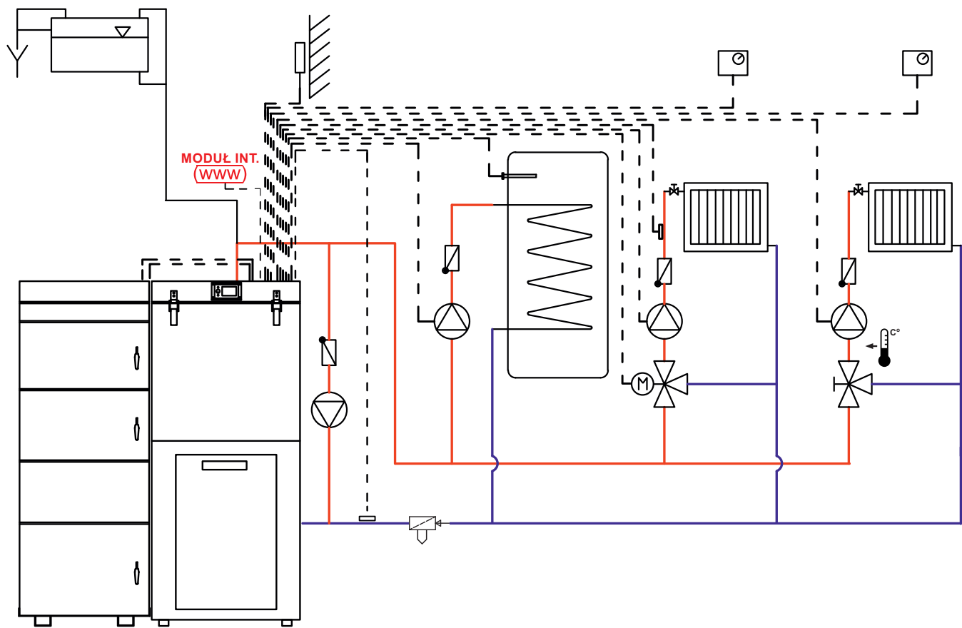
Przykładowy schemat obrazuje możliwość wykorzystania automatyki do sterowania instalacją. Schemat nie stanowi projektu instalacji.
